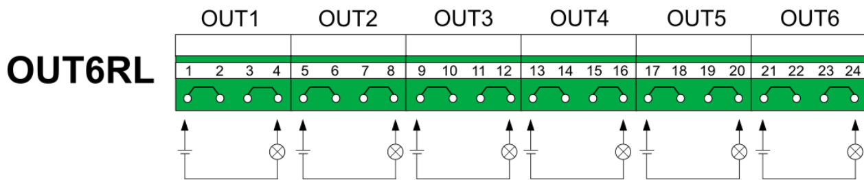
Rys. 6.17 Schemat podłączeń dla modułu OUT6RL.
