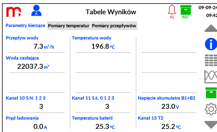
Rys. 11.3 Przykładowy wygląd okna Tabele Wyników.
