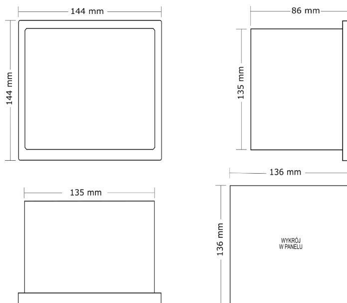
Rys. 5.1 Wymiary obudowy urządzenia DL5 oraz wymiary wykroju w panelu.
