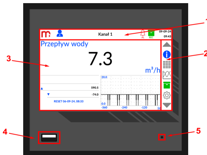
Rys. 7.1 Panel przedni urządzenia.
