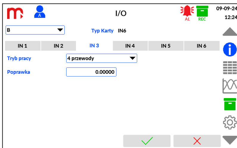
Rys. 12.2 Przykładowy wygląd okna ustawień Wejść i Wyjść - I/O.
