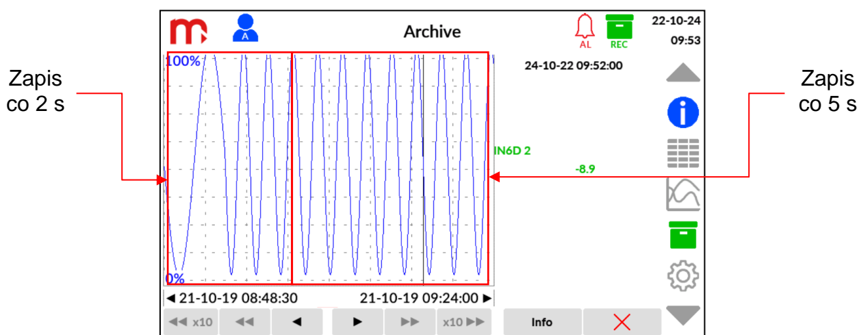
Rys. 11.12 Przykładowy wygląd okna podglądu archiwum – zmiana częstości zapisu do archiwum.
