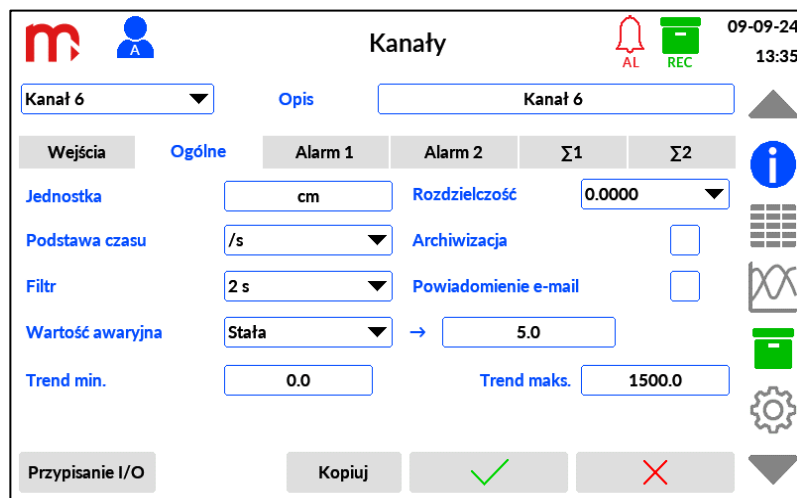
Rys. 12.5 Przykładowy wygląd okna ustawień ogólnych kanału - Kanały.
