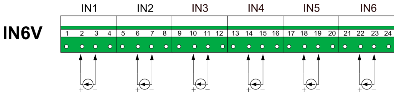
Rys. 6.8 Schemat podłączeń dla modułu IN6V.
