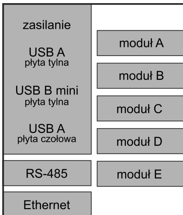
Rys. 3.2 Separacja galwaniczna w urządzeniu DL5 (separacja funkcjonalna 500VAC @ 1min)
