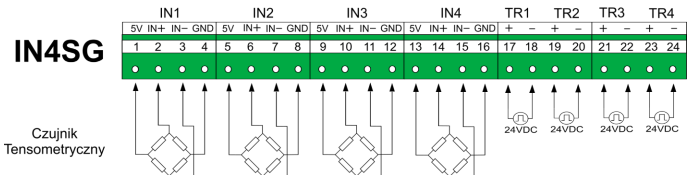
Rys. 6.12 Schemat połączeń dla modułu IN4SG.
