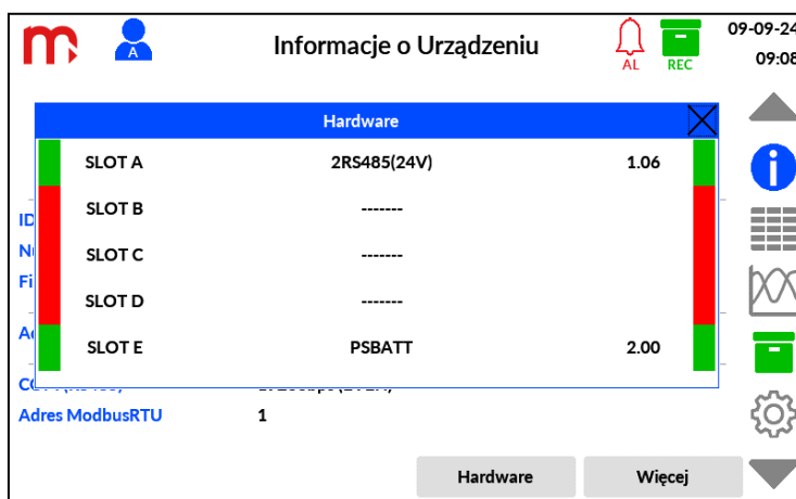
Rys. 11.2 Hardware – okno informujące o konfiguracji hardware.
