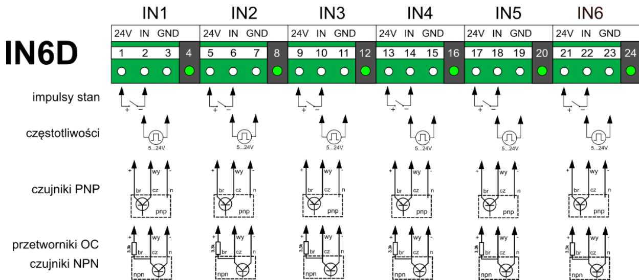
Rys. 6.13 Schemat połączeń dla modułu IN6D.
