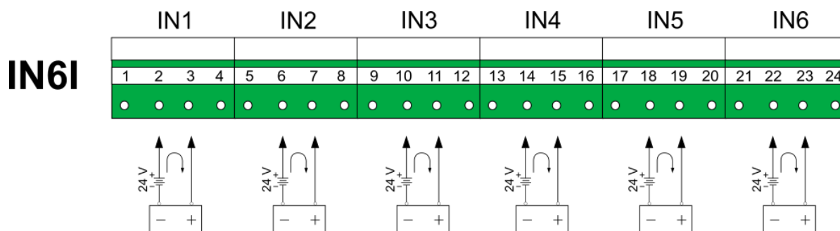
Rys. 6.4 Schemat połączeń dla modułu IN6I.
