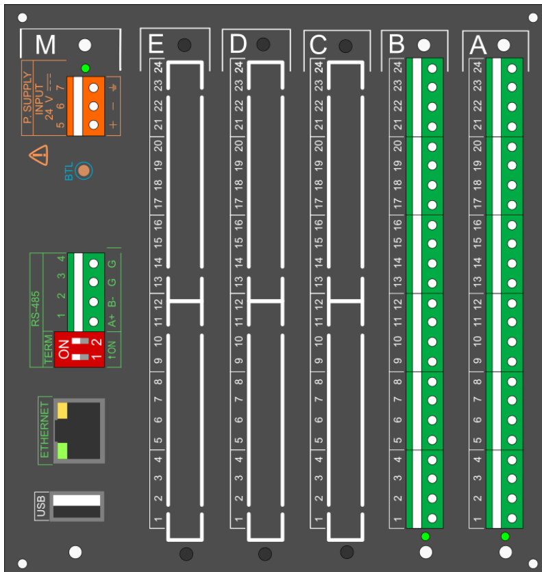
Rys. 6.1 Przykładowy widok płyty tylnej DL5.
