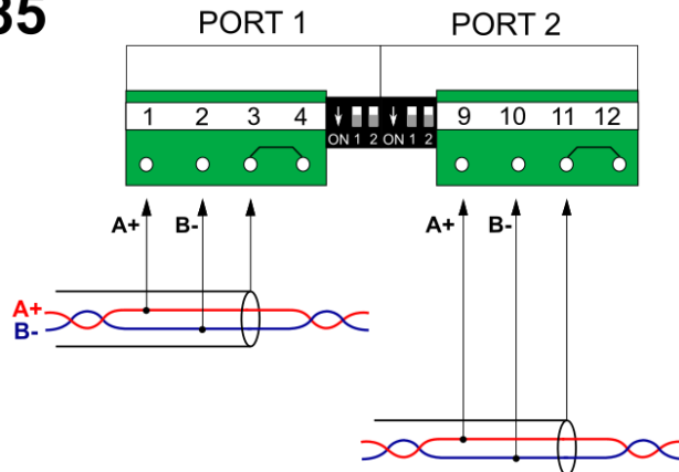
Rys. 6.15 Schemat podłączeń dla modułu 2RS485.
