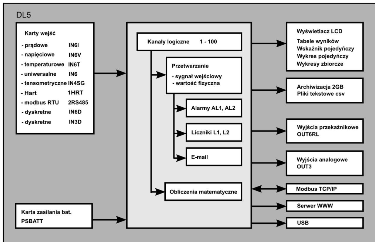
Rys. 3.1 Schemat blokowy DL5
