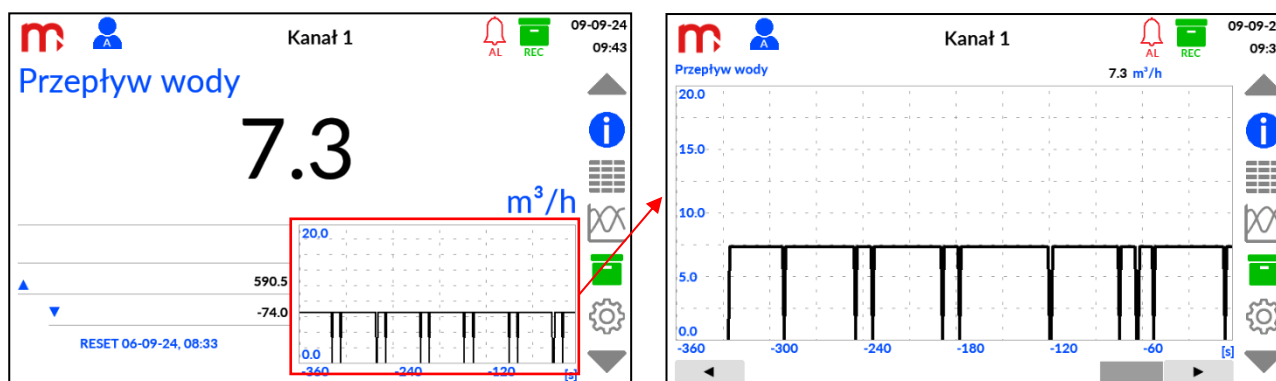
Rys. 11.6 Naciśnięcie obszaru trendu w oknie pojedynczego wyniku powoduje powiększenie wykresu na cały ekran.
