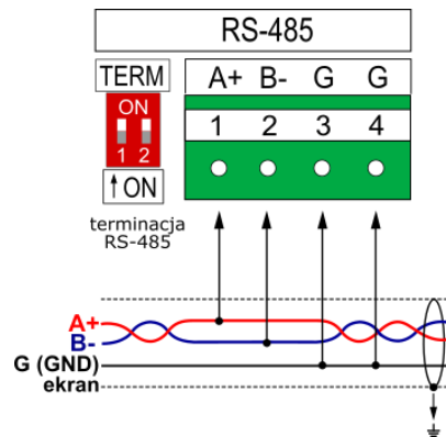
Rys. 6.22 Schemat podłączenia RS-485.
