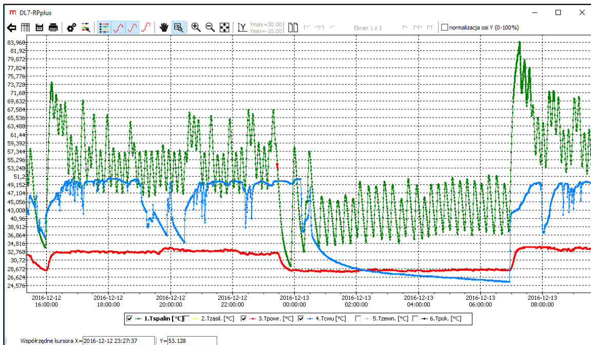
Rys. 3.3 Okno wykresów.
